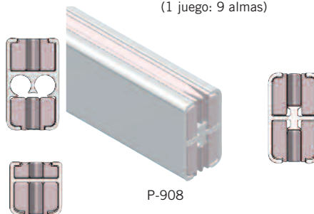
ALMAS PARA CURVAR PERFILES 908 (1 juego: 9 almas)
