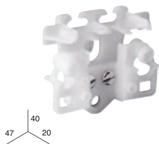
CORREDERA MAESTRA CON RUEDA
