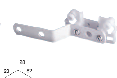
CORREDERA MAESTRA CON RUEDA Y PATA CORTA (recomendada para riel con curva)
