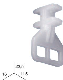
FIJADOR INTERMEDIO
