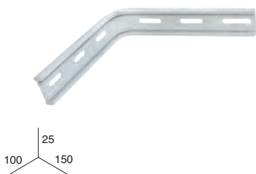
SOPORTE DE PERFIL DE ALUMINIO 15 cm. BASE LARGA
