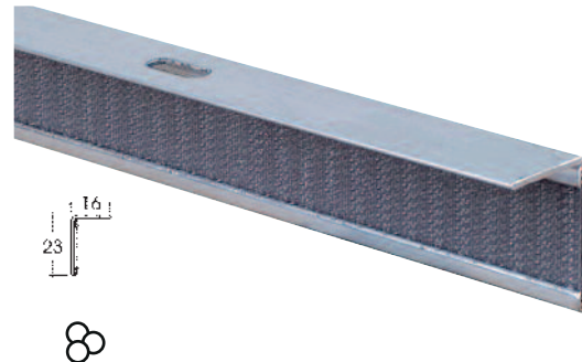
PERFIL 7198 (CON CINTA GANCHO)
