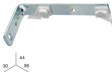
SOPORTE DOBLE 3-9 cm.
