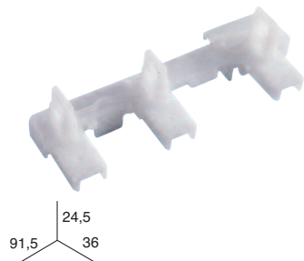
TERMINAL IZQUIERDA Y DERECHA
