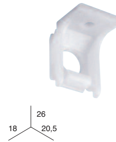
ESTRIBO
