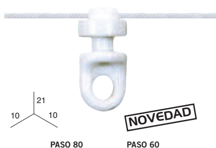
CORREDERA CON HILO "CHYC"
