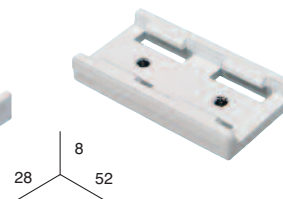
EMPALME
