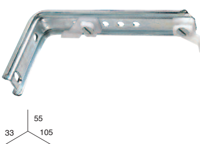
SOPORTE DOBLE REFORZADO 3-9 cm.
