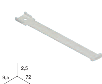
DISTANCIADOR 6 cm.
