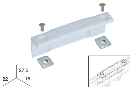
UNIÓN MANGUITOS PORTA-POLEAS P-900 Y 910 (para porta-poleas 7297060 y 7298060)
