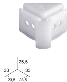
UNIÓN ESQUINA TECHO, PARED
