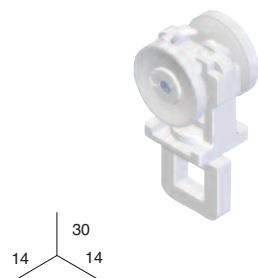
CORREDERA CON EJE ROTATIVO
