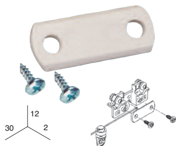
PUENTE PARA CORREDERA MAESTRA (recomendado para corredera con hilo)
