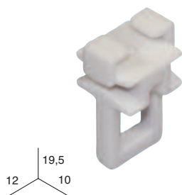
CORREDERA SIMPLE (Siempre junto al distanciador)
