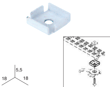
SUPLEMENTO PARA SOPORTES
