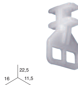
FIJADOR INTERMEDIO
