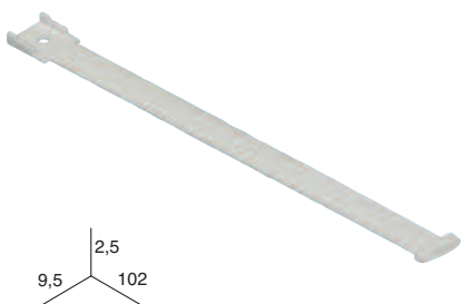
DISTANCIADOR 9 cm.
