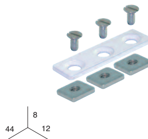
PLETINA UNIÓN CRUZ
