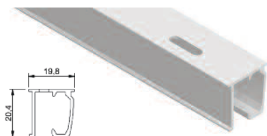
PERFIL 7700 DE 6,00 m.
