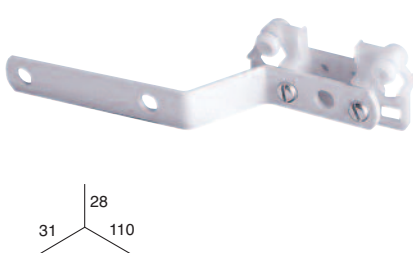
CORREDERA MAESTRA CON RUEDA Y PATA
