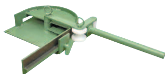
MÁQUINA PARA CURVAR PERFIL DE ALUMINIO (Con almas para curvar)
