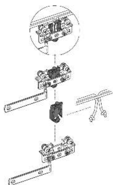
BRIDA CORDÓN
