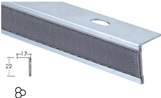
PERFIL 1076 (CON CINTA GANCHO)
